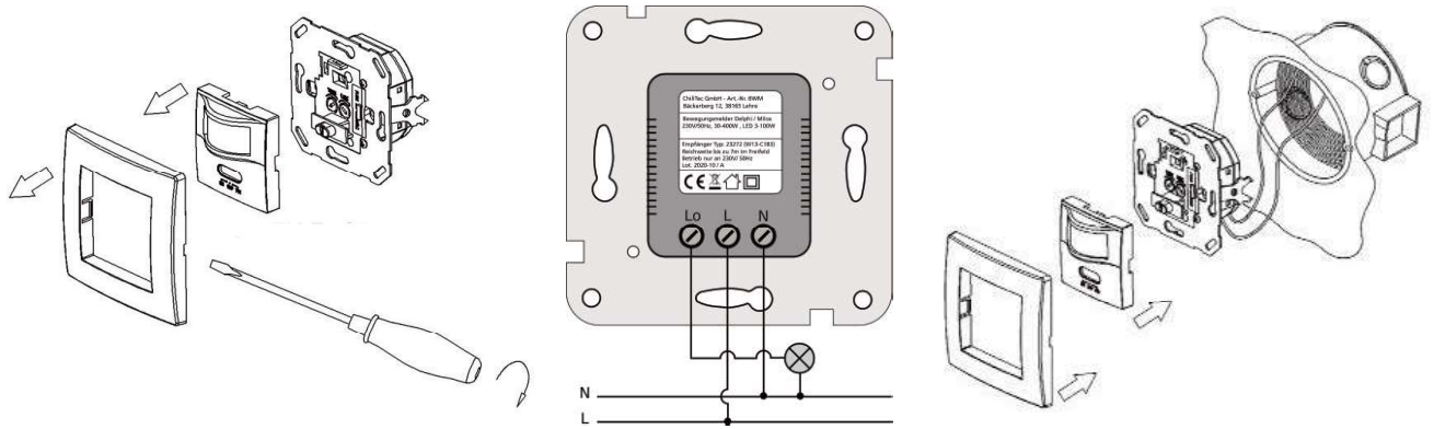
Bewegungsrichtung immer parallel zum Sensor
